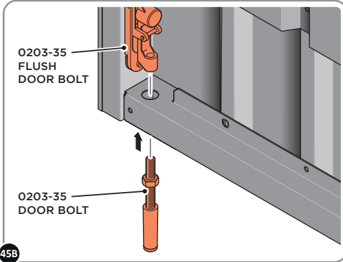
45B ATTACH DOOR BOLT ONTO FLUSH DOOR BOLT.
